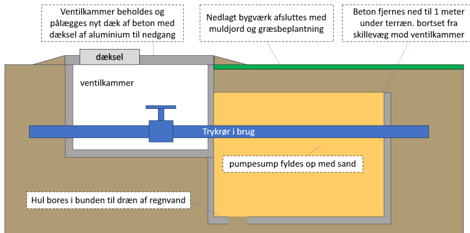
Figur 3 – Forventet ombygning
