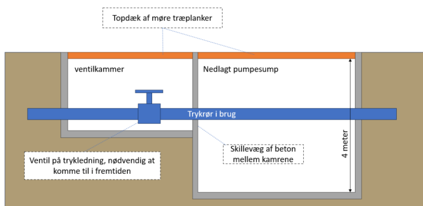
Figur 2 – nuværende konstruktion
