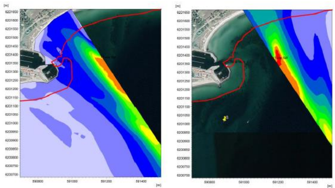
Figur 2-3. Færgens genererede bølger samt 3 meter kontur. Øverst: Tunø Røn – Tunø mole. Fart = 10 knob, nederst: Sælvig N – Tunø SØ. Fart = 29,5-10 knob.
