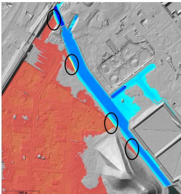
Fig. 3. Modtaget fra ansøger. Terrænhævning (markeret med sorte ringe), oversvømmelse fra Harrestrup Å ved vandstand på kote 1,85 m DVR90 uden terrænhævning (rød) og efter terrænhævning (blå). De er kun de to terrænhævninger nederst i figuren, der ansøges om her.
