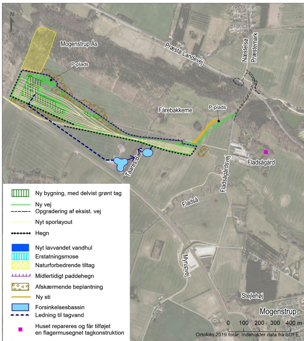
Figur nr. 1 Der viser placering og indretning af værkstedsfaciliteterne på det ca. 70 hektar store areal
