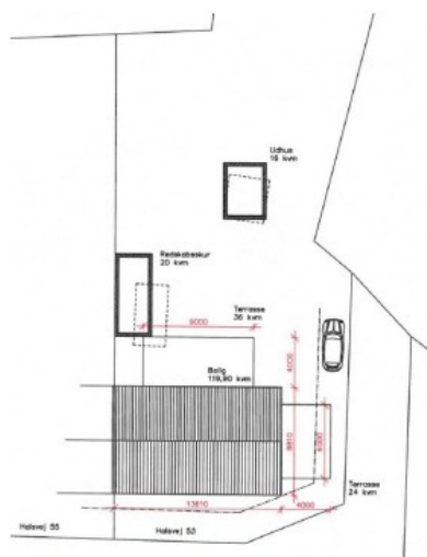
Situationsplan for den ny bebyggelse
