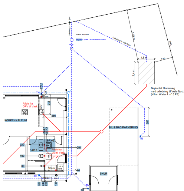
Kloakplan – rød er husspildevand
