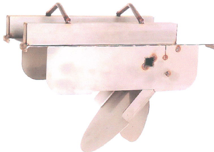
Wavin rottespærre (indsatsmodel til lige gennemløb)
