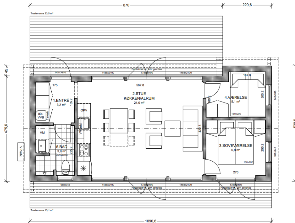
Grundplan nyt sommerhus – under: situationsplan (eksisterende vist grå)
